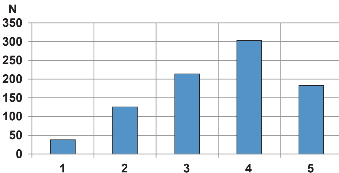
Résistance comparative au déchirement des différentes épaisseurs 1 : 0.8mm ; 2 : 1.6mm ; 3 : 2.3mm ; 4 : 3.2mm ; 5 : 2.3mm avec grille en acier inoxydable
