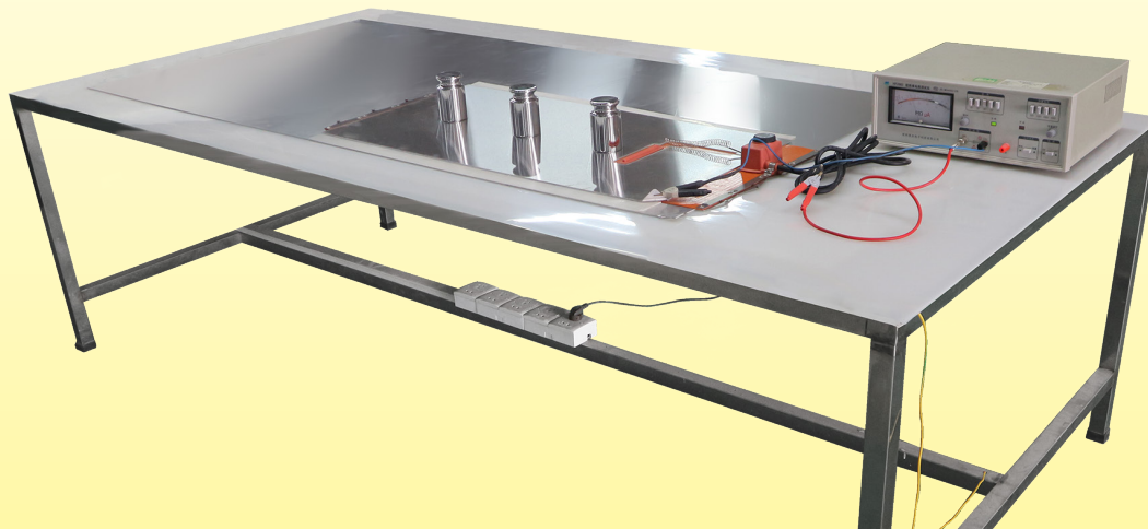
Dispositif de mesure de la résistance d'isolement. Les valeurs mesurées sont toujours supérieures à 0.1Gohm
